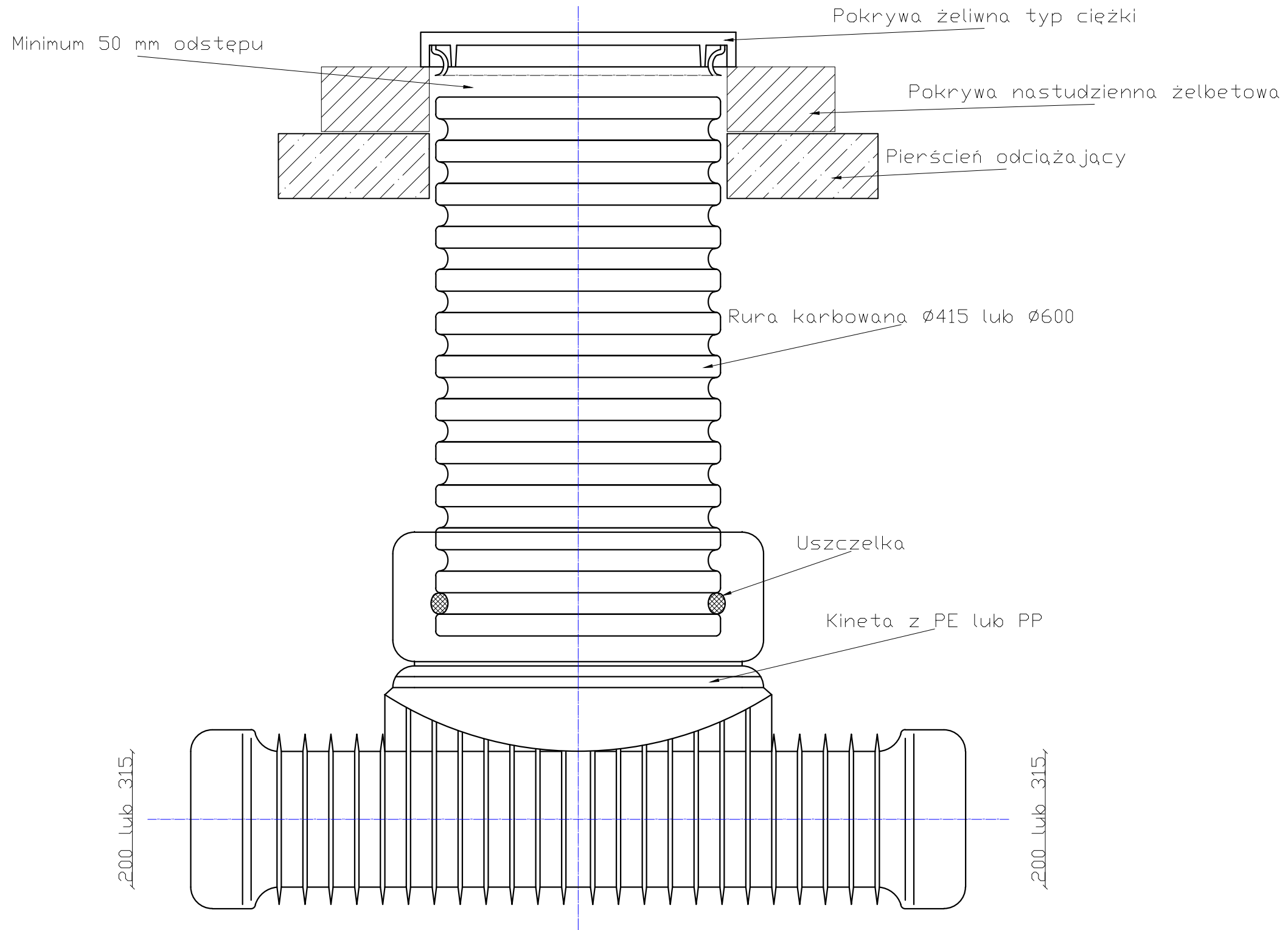
Studzienka \varnothing 415 lub \varnothing 600 z pokrywą żeliwną
